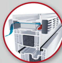
GECCO 4 zárva
