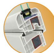
6 kamrás rendszer síkban félig eltolt szárny
